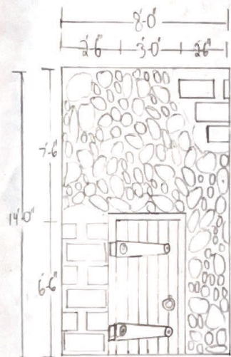
E ELEVATION
