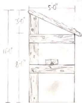
J ELEVATION
