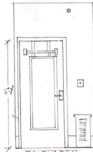
② ELEVATION
